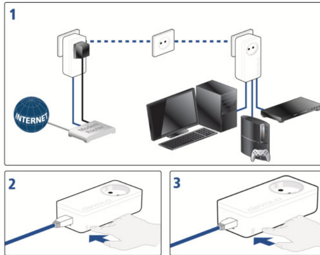
Abb. 4 dLAN-Verschlüsselung mittels des Verschlüsselungstasters aufbauen
